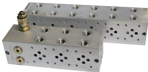
Blocs forés 1 à 12 postes Avec ou sans LP
