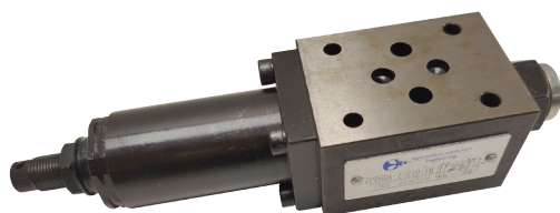
Valves modulaires CETOP 3 et 5 Clapets, valves d'équilibrage Limiteurs de pression Limiteurs de débit
